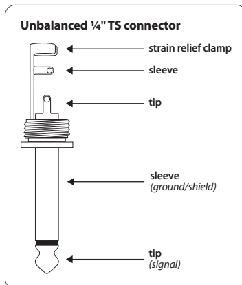
Bild 3.2: 6,3-mm-monojack
