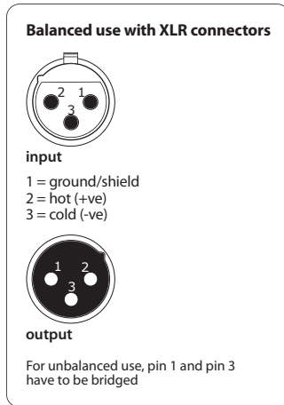
Bild 3.1: XLR-förbindelser
