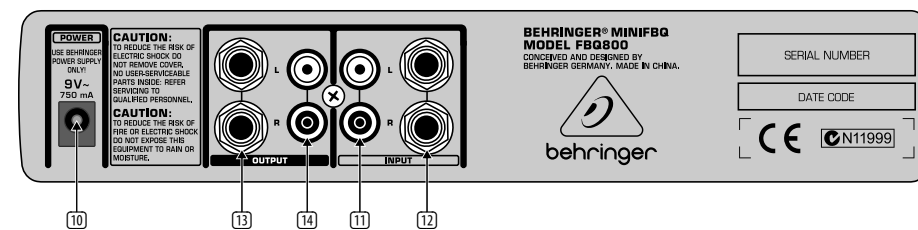
Panel trasero del FBQ800
