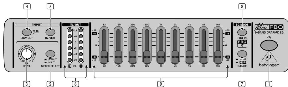
Face avant du FBQ800
