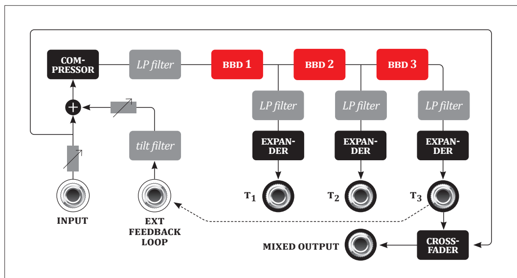
fig. 1: SARAJEWO BLOCK DIAGRM
